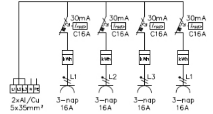
Kaaviokuva: FipaX0400MV4 pääkaavio
